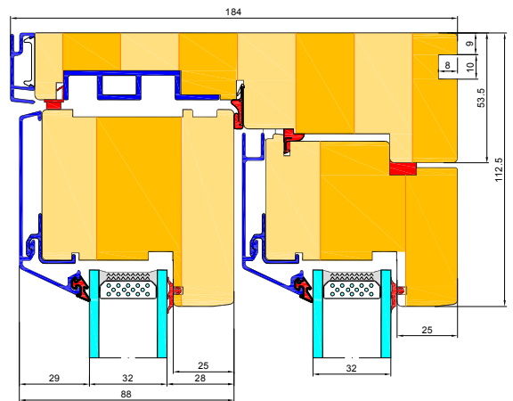
A-A B-B
