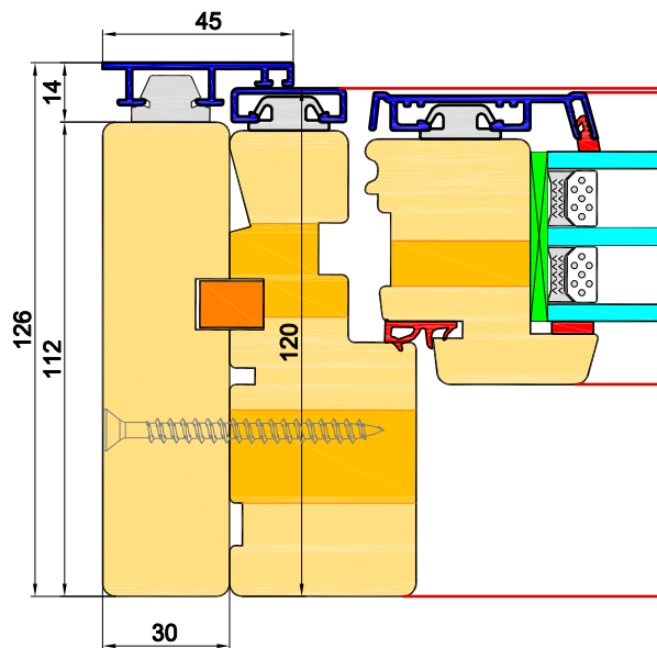
Stockverbreiterung 30mm
