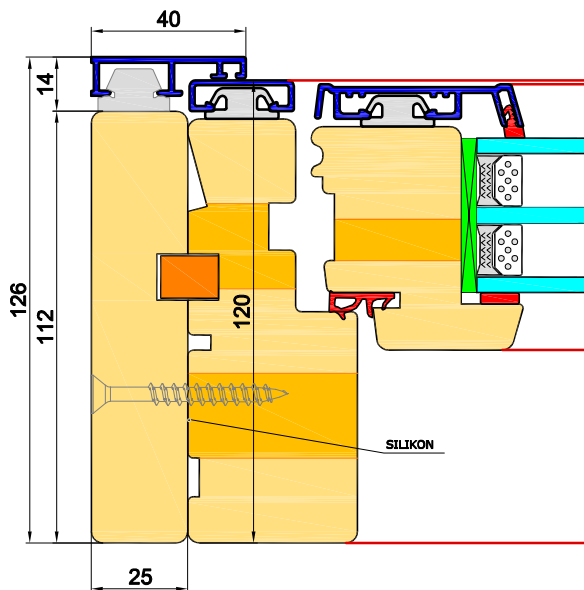
Stockverbreiterung 25mm
