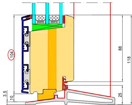
glasfaser schwelle
