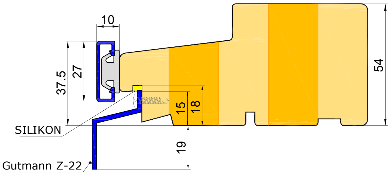
Aluminiumfensterbank _ Gutmann Z-22
