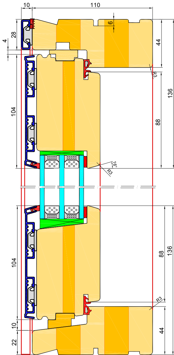
hölzerne schwelle
