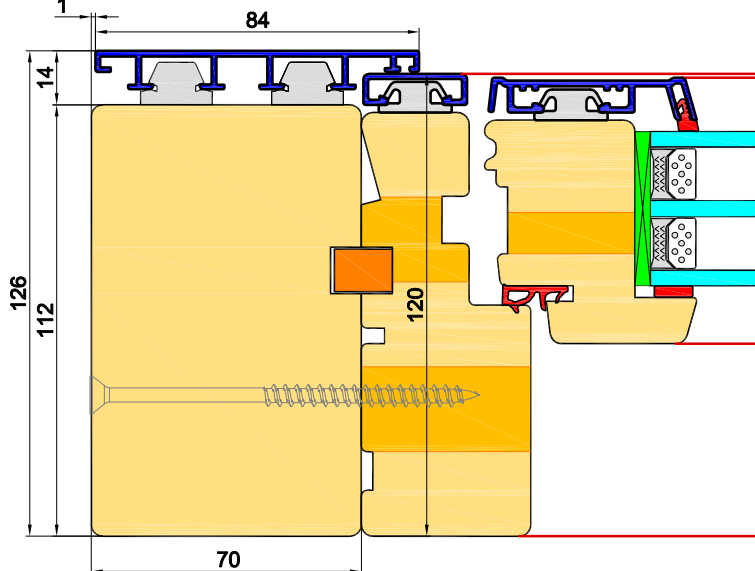
Stockverbreiterung 70mm
