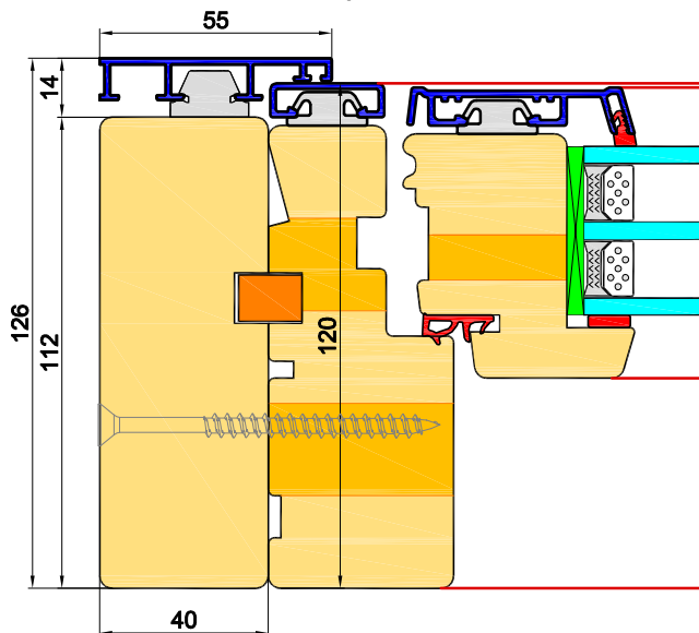
Stockverbreiterung 40mm
