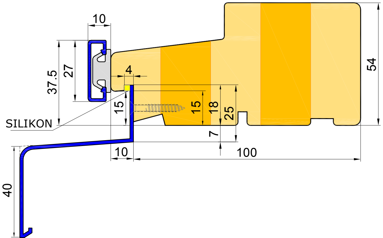
Aluminiumfensterbank _ ALURON
