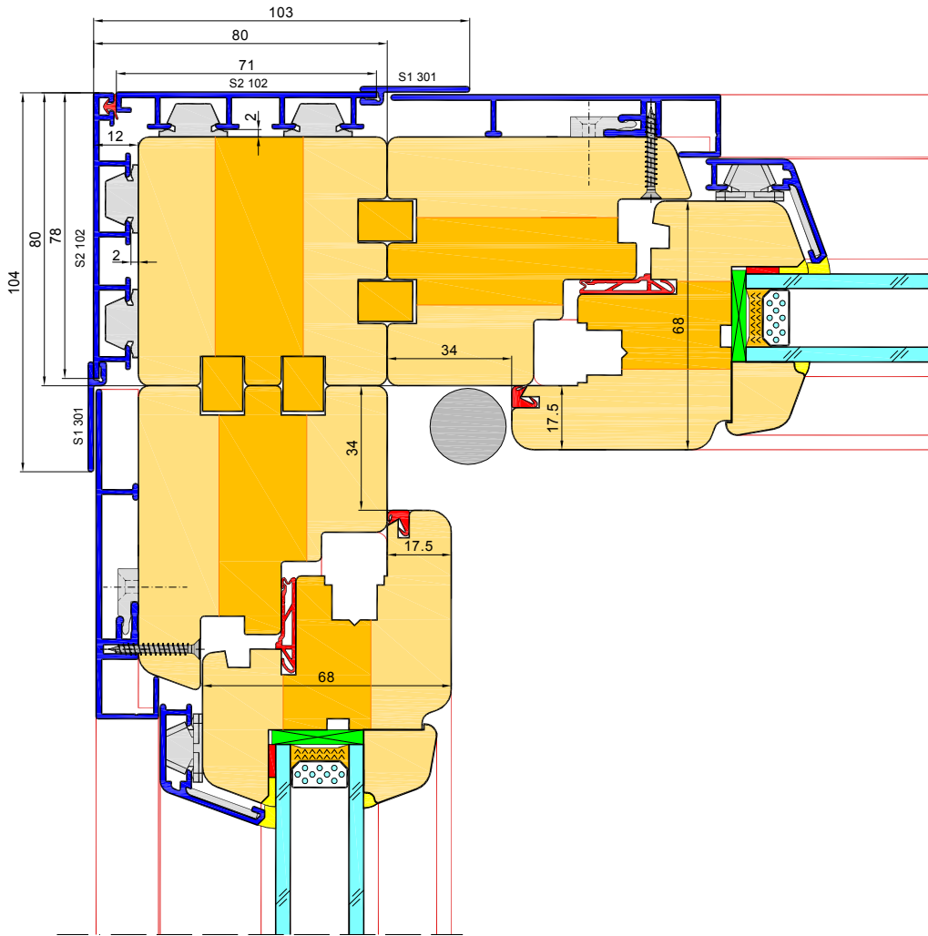
Kopplung 90°
