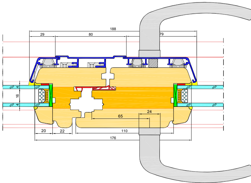
2 fl. Balkontür mit Stulp
